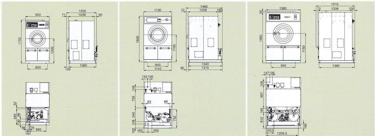
外形寸法図
