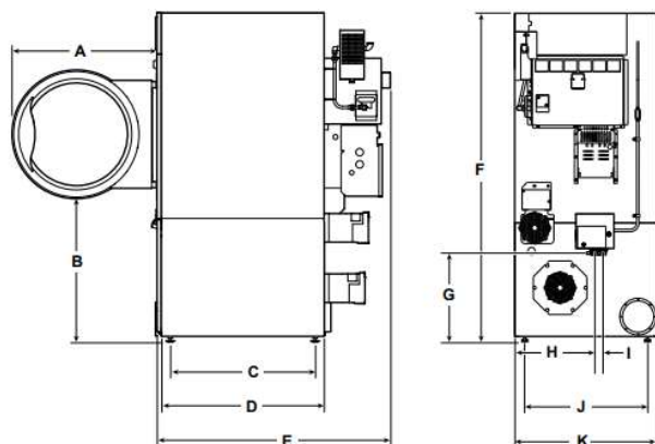
UU-030 寸法図
