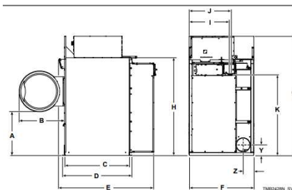
UU-200 寸法図
