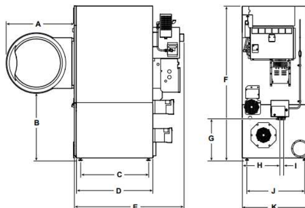
UU-035 寸法図
