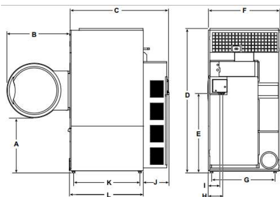
UU-050 寸法図
