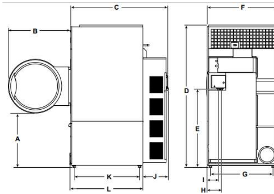
UU-075 寸法図
