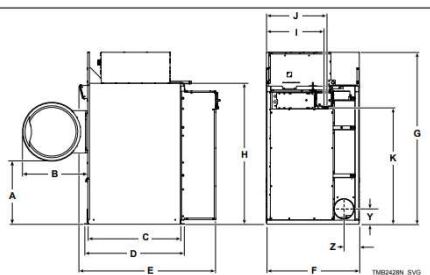
UU-120 寸法図
