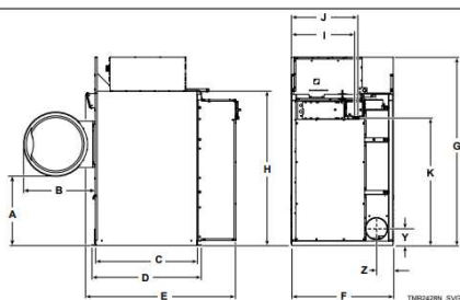
UU-170 寸法図
